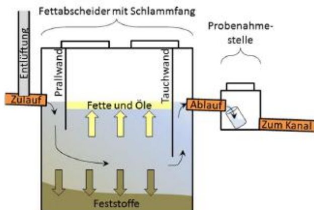
Abbildung 1: Schematische Darstellung eines Fettabscheiders mit Probenahmestelle
